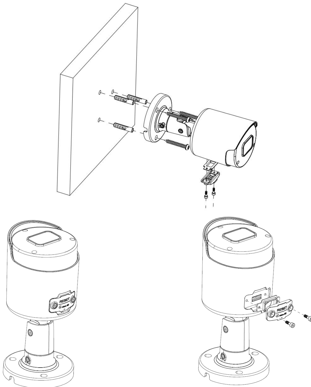
Рисунок 2. Монтаж камеры
