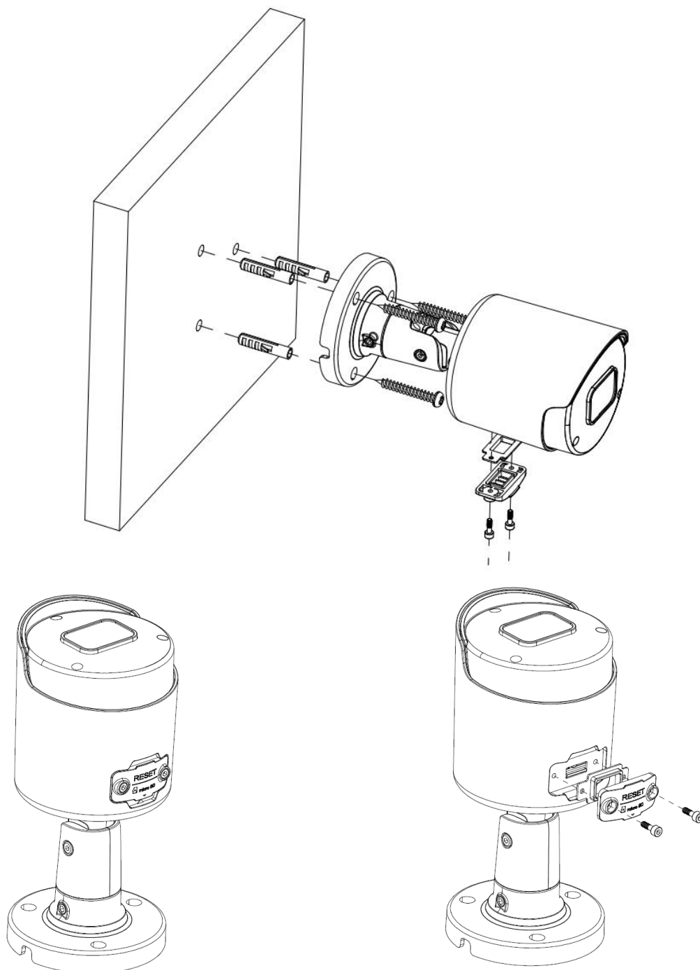
Рисунок 2. Монтаж камеры
